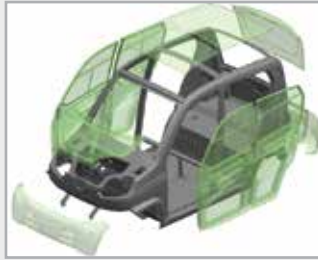
MONOCOQUE BODY
